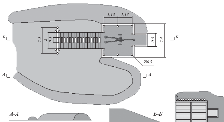
Рис. 8. Укрытие для пушки Pak-38 и прислуги (план и разрезы по А-А и Б-Б)
