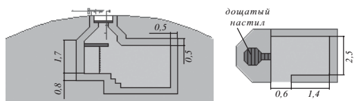
Рис. 16. Универсальное железобетонное сооружение (разрез и план)
