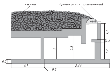
Рис. 5. Универсальный железобетонный ДОТ в стиле «линии Маннергейма» (план и разрез по А-А)
