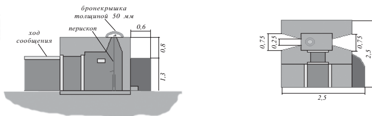
Рис. 15. Железобетонный наблюдательный пункт (разрез и план)
