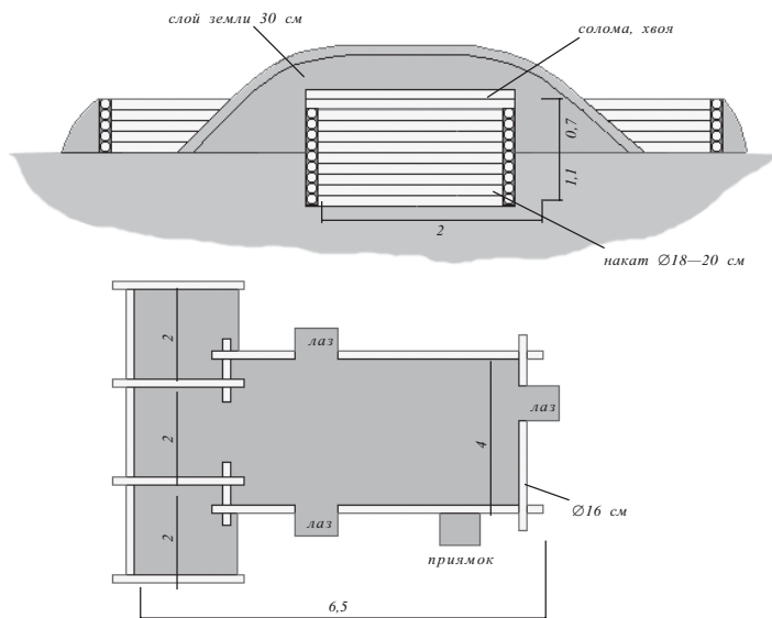
Рис. 17. Огневая точка — блиндаж (разрез и план)
