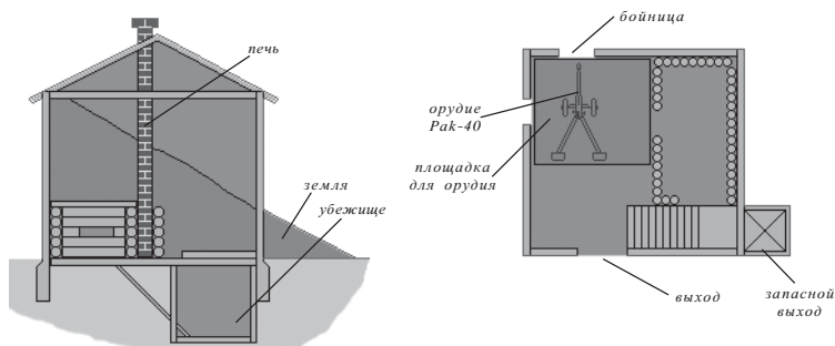
Рис. 10. Противотанковая огневая точка в стрелочном железнодорожном домике (разрез и план)
