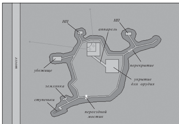
Рис. 23. Немецкий окоп для противотанковой пушки Pak-40
