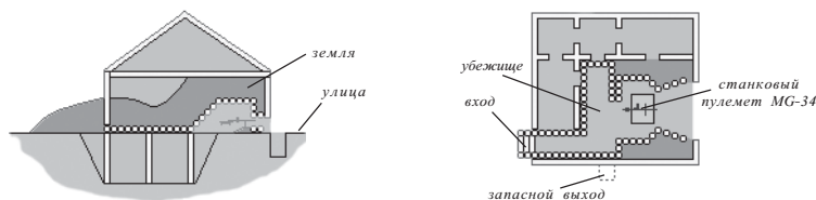
Рис. 11. Немецкая пулеметная огневая точка с помещением для команды (разрез и план)
