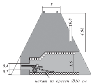
Рис. 9. Позиция для пушки Pak-40 в железнодорожной насыпи
