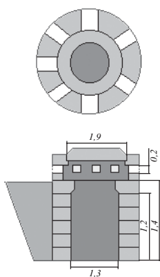
Рис. 6. Немецкий железобетонный блокгауз (план и разрез)
