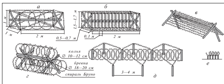
Рис. 3. Противопехотные проволочные препятствия немецкой обороны:
