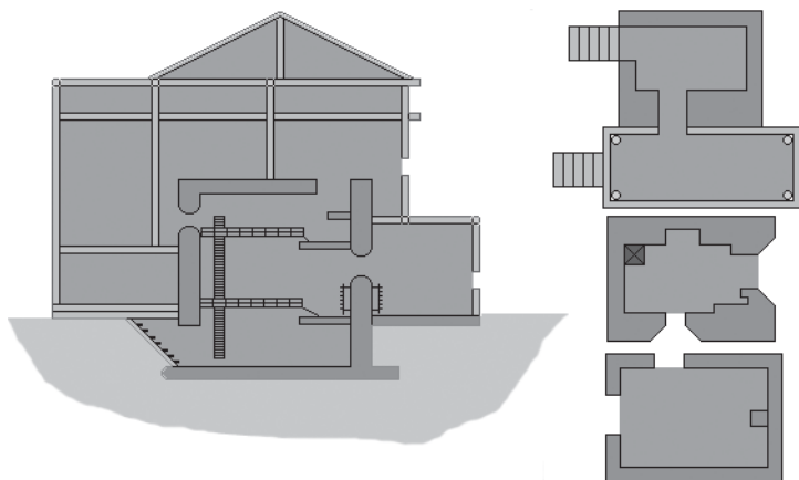
Рис. 14. Железобетонный наблюдательный пункт в деревне Доры (разрез и поэтажные планы)
